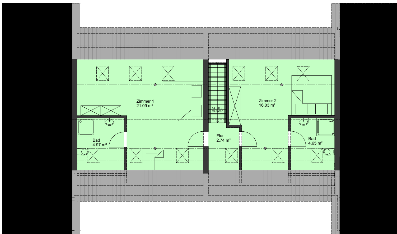
Grundriss Dachgeschoss Wohnung
